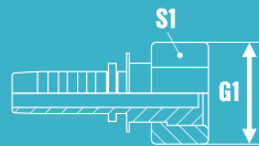
METRISCHE KOPPELING
