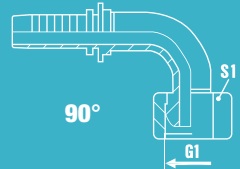
PIJPOPNAME 22L
