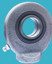
GELENKOOG (ENGELSMODEL)
