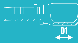
BANJO KOPPELING
