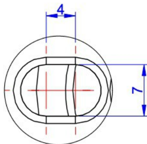
細部放大圖 A 比例 2 : 1
